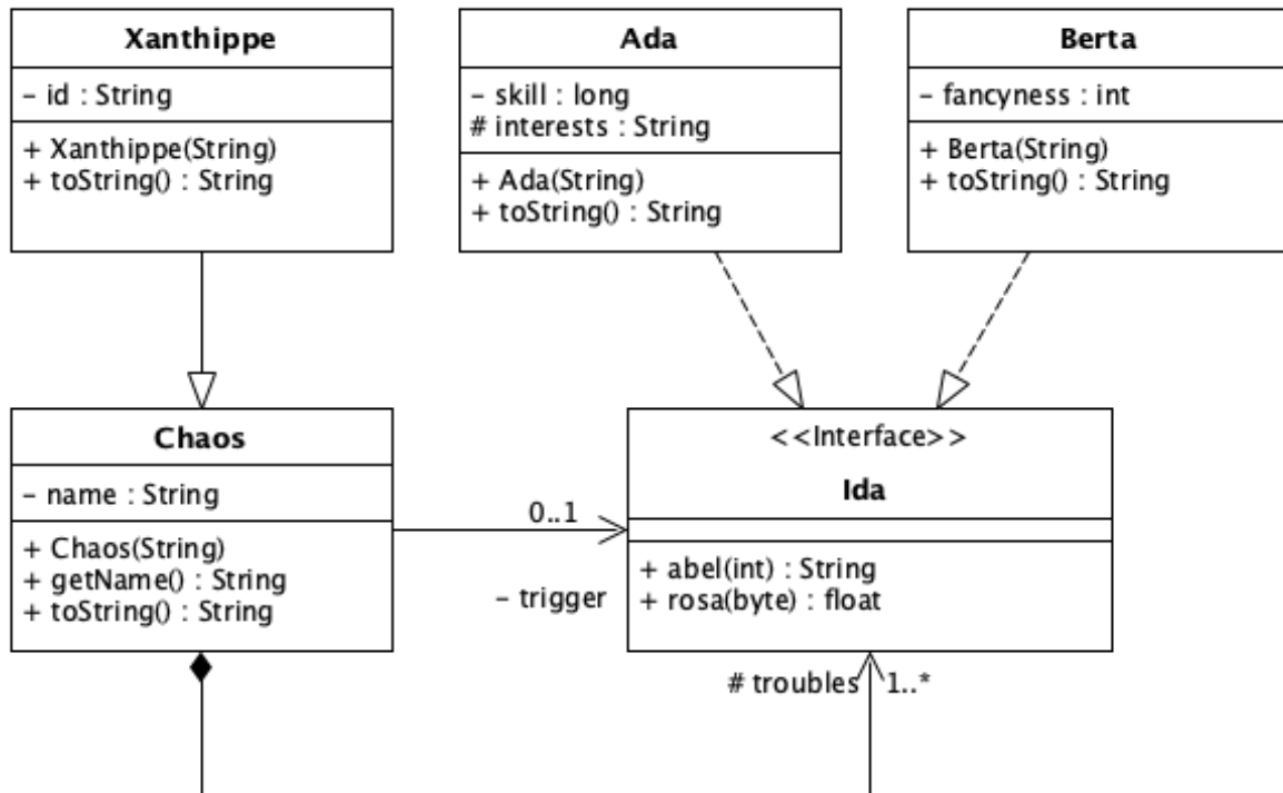
Abbildung 7.8: UML
