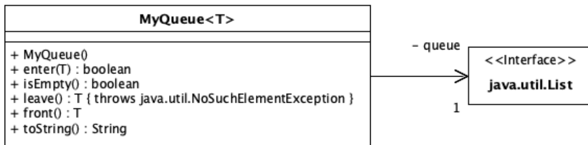
Abbildung 8.1: UML
