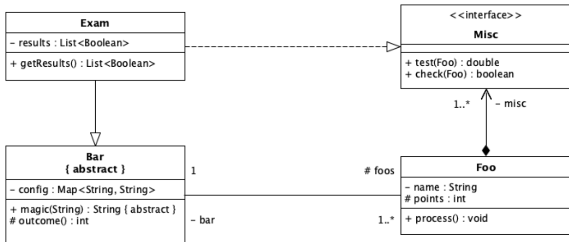
Abbildung 7.5: UML
